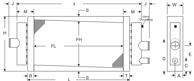
Figure 4 - DA, LA Dimension Info
